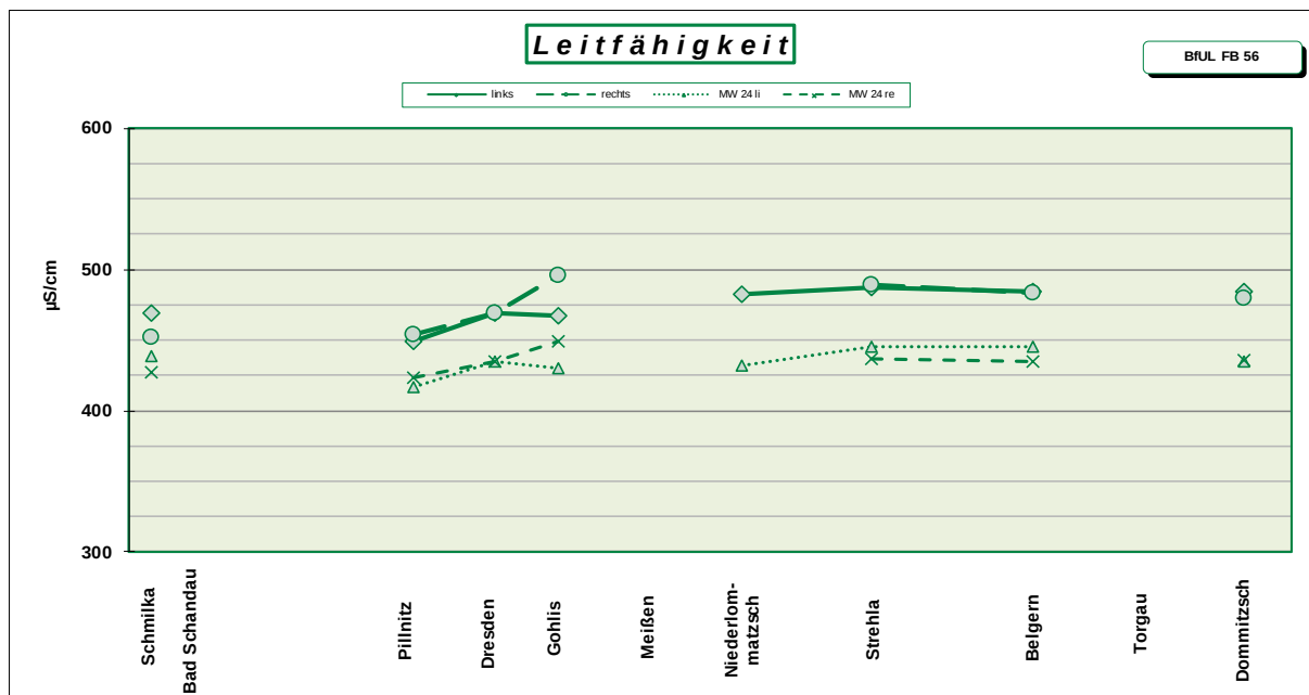
Abb. 2: Leitfähigkeit in \mu\text{S}/\text{cm} der Einzelmessungen April 2025 (links, rechts) und dem Jahresmittelwert 2024 (MW 24 li, re)
