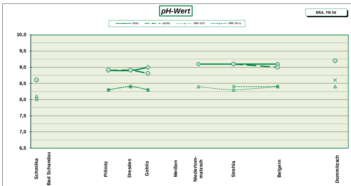
Abb. 3: pH-Werte aus den Einzelmessungen April 2025 (links, rechts) und dem Jahresmittelwert 2024 (MW 24 li, re)
