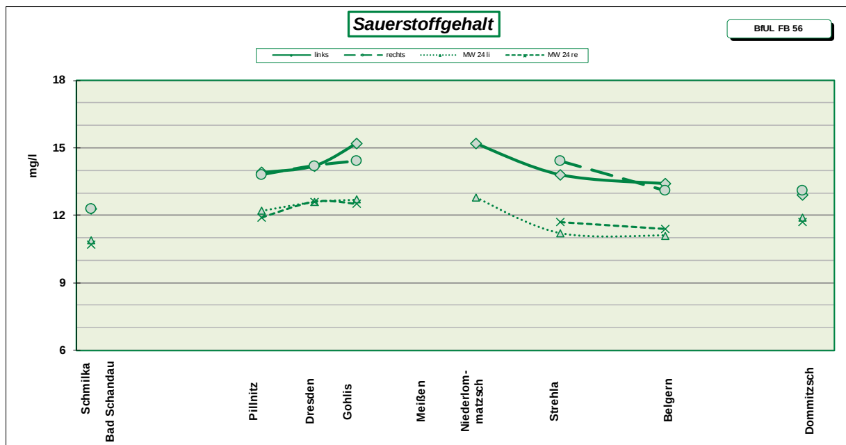
Abb. 1: Sauerstoffgehalt in mg/l der Einzelmessungen April 2025 (links, rechts) und dem Jahresmittelwert 2024 (MW 24 li, re)
