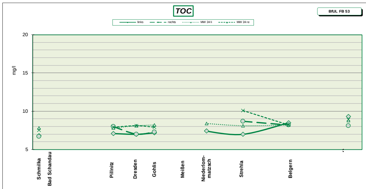
Abb. 4: TOC in mg/l der Einzelmessungen April 2025 (links, rechts) und dem Jahresmittelwert 2024 (MW 24 li, re)
