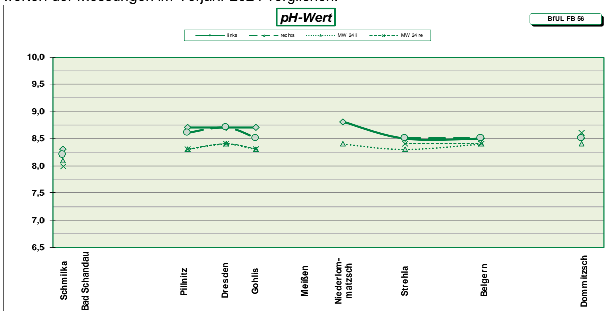
Abb. 3: Mittelwerte der pH-Werte aus den Messungen März 2025 (links, rechts) und März 2024 (MW 24 li, re)
