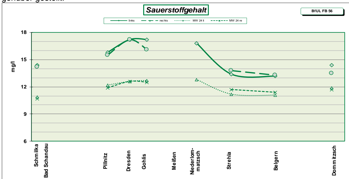
Abb. 1: Mittelwerte des Sauerstoffgehalts in mg/l aus den Messungen März 2025 (links, rechts) und März 2024 (MW 24 li, re)
