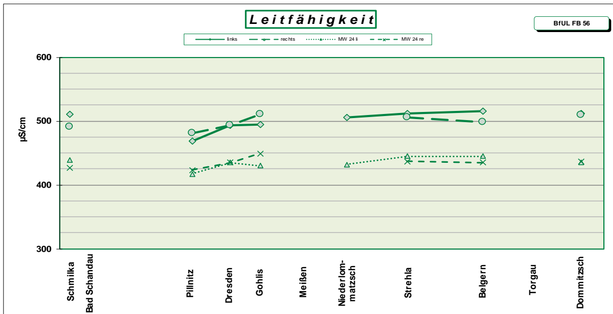
Abb. 2: Mittelwerte der Leitfähigkeit in µS/cm aus den Messungen März 2025 (links, rechts) und März 2024 (MW 24 li, re)
