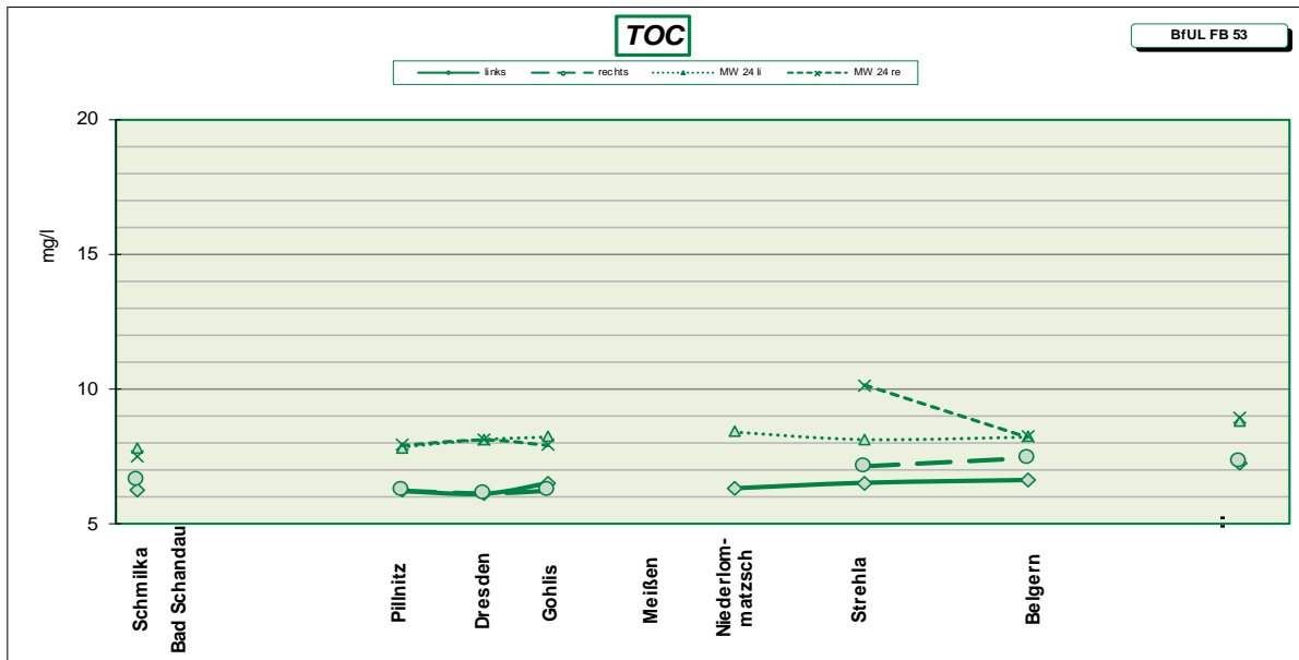
Abb. 4: Mittelwerte des TOC in mg/l aus den Messungen März 2025 (links, rechts) und März 2024 (MW 24 li, re)
