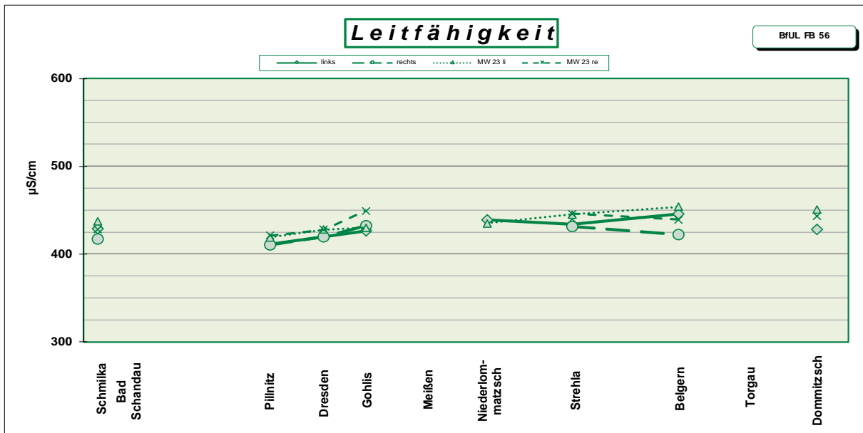
Abb. 2: Mittelwerte der Leitfähigkeit in \mu\text{S}/\text{cm} aus den Messungen November 2024 (links, rechts) und November 2023 (MW 23 li, re)
