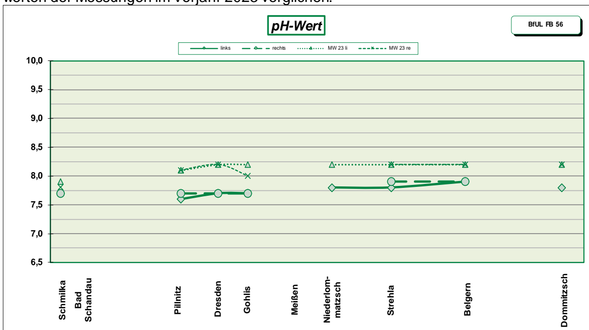
Abb. 3: Mittelwerte der pH-Werte aus den Messungen November 2024 (links, rechts) und November 2023 (MW 23 li, re)
