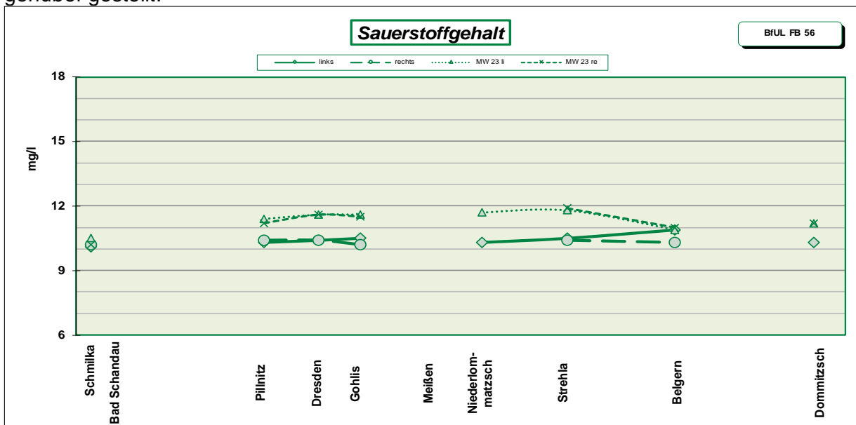
Abb. 1: Mittelwerte des Sauerstoffgehalts in mg/l aus den Messungen November 2024 (links, rechts) und November 2023 (MW 23 li, re)
